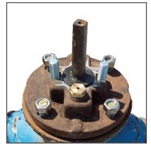
Stopfbüchse umrüsten
